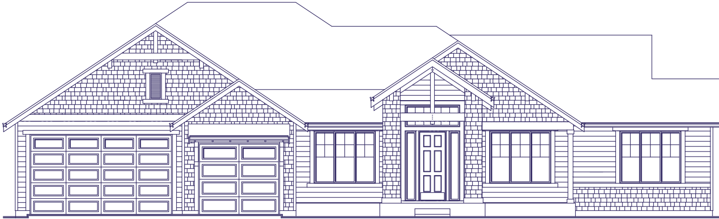
ELEVATION A
